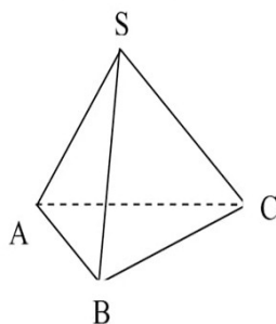
Hình chóp tam giác S.ABC (Tứ diện S.ABC)
