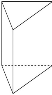
Lăng trụ đứng
