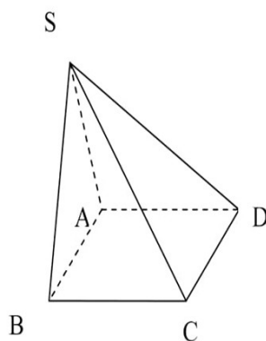
Hình chóp tứ giác S.ABCD
