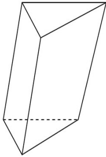
Lăng trụ thường
